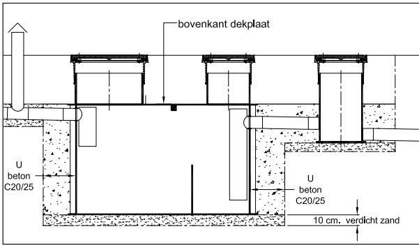
Afbeelding 6. Aanvullen met beton tot bovenkant dekplaat
